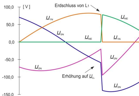
Bild 01 Spannungsverlauf vor und nach einem Erdschluss
