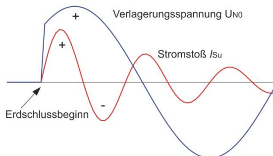
Bild 04 Verlagerungsspannung und Stromstoß
