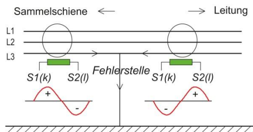
Bild 05 Ortsbestimmung des Erdschlusses
