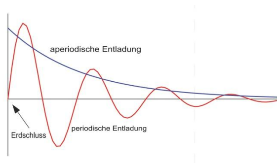
Bild 02 Typische Verläufe des Entladestromes
