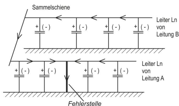
Bild 03 Richtung des Entladestromes
